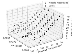
(b) Modelo de Greenberg en el carril 5.
