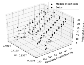
(a) Modelo de Greenshield en el carril 4.
