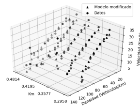
(d) Modelo de Drake en el carril 4.
