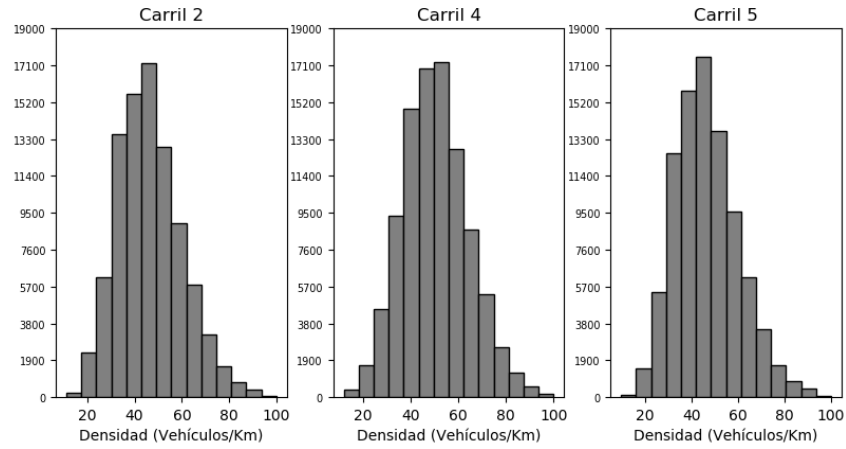
Figura 1: Frecuencias de las densidades en los diferentes carriles.
