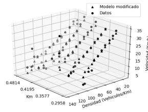
(f) Modelo de Pipes en el carril 4.
