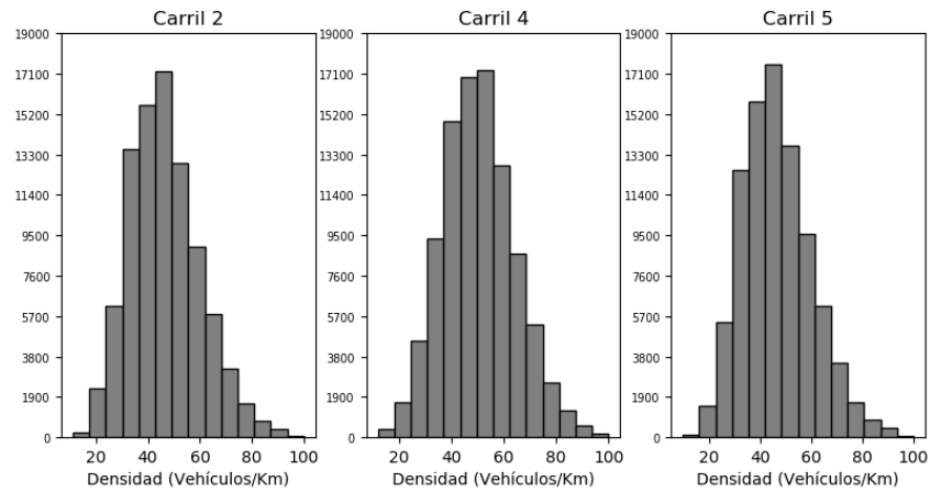
Figura 2: Frecuencias de las velocidades en los diferentes carriles.
