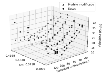
(g) Modelo de MacNicholas en el carril 2.
