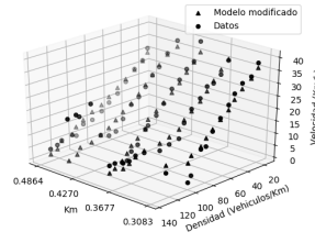
(f) Modelo de Pipes en el carril 5.
