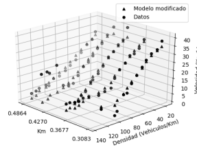
(d) Modelo de Drake en el carril 5.
