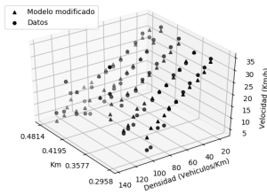
(e) Modelo de Drew en el carril 4.
