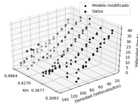
(e) Modelo de Drew en el carril 5.
