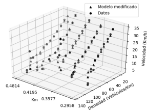
(g) Modelo de Nicholas en el carril 4.
