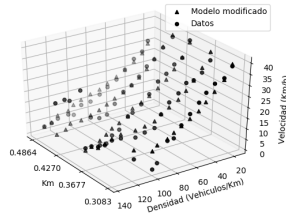
(a) Modelo de Greenshield en el carril 5.
