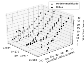
(c) Modelo de Underwood en el carril 5.
