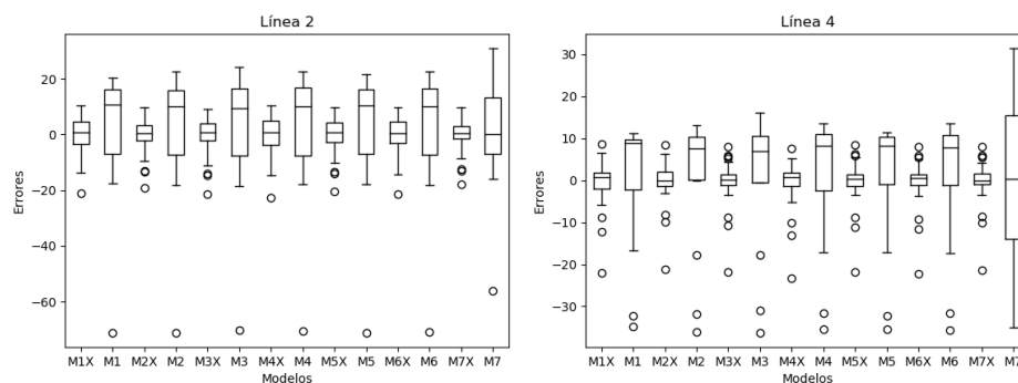
(a) Comparación de los errores en el carril 2. (b) Comparación de los errores en el carril 4.
