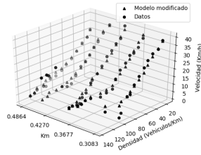
(g) Modelo de Nicholas en el carril 5.
