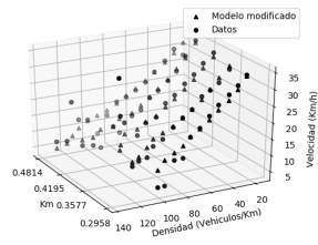
(c) Modelo de Underwood en el carril 4.
