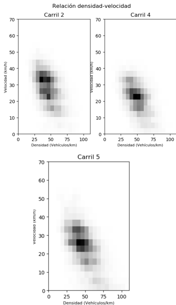
Figura 4: Frecuencias de las parejas de densidad y velocidad. Los puntos más oscuros indican frecuencias grandes.
