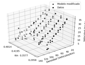
(b) Modelo de Greenberg en el carril 4.
