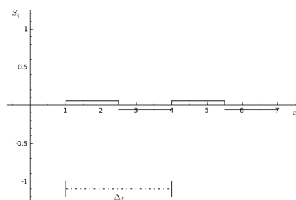
(d) S_4(x) .
