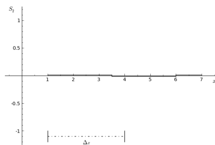
(b) S_2(x) .
